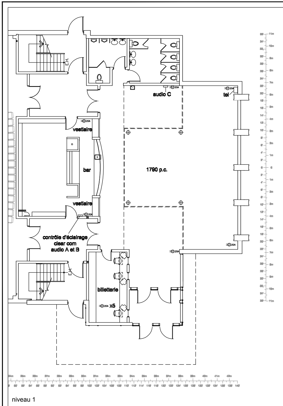
plan du foyer
