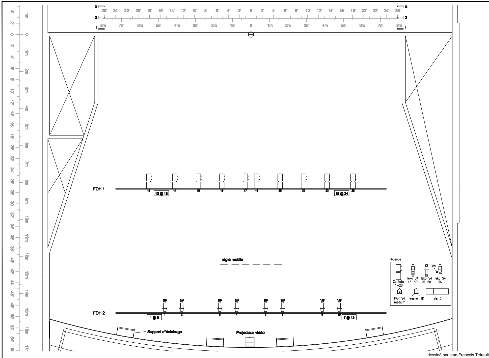
plan d'éclairage FOH
