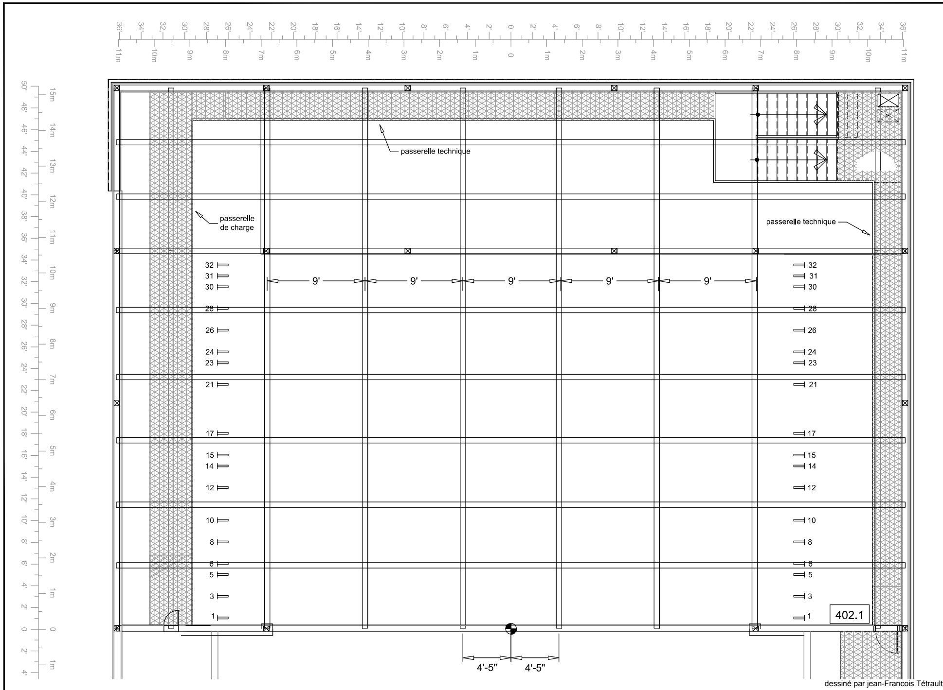
plan de scène - plafond
